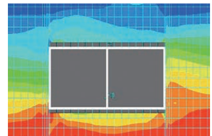
免震地下構造物 Seismic isolation underground structure
